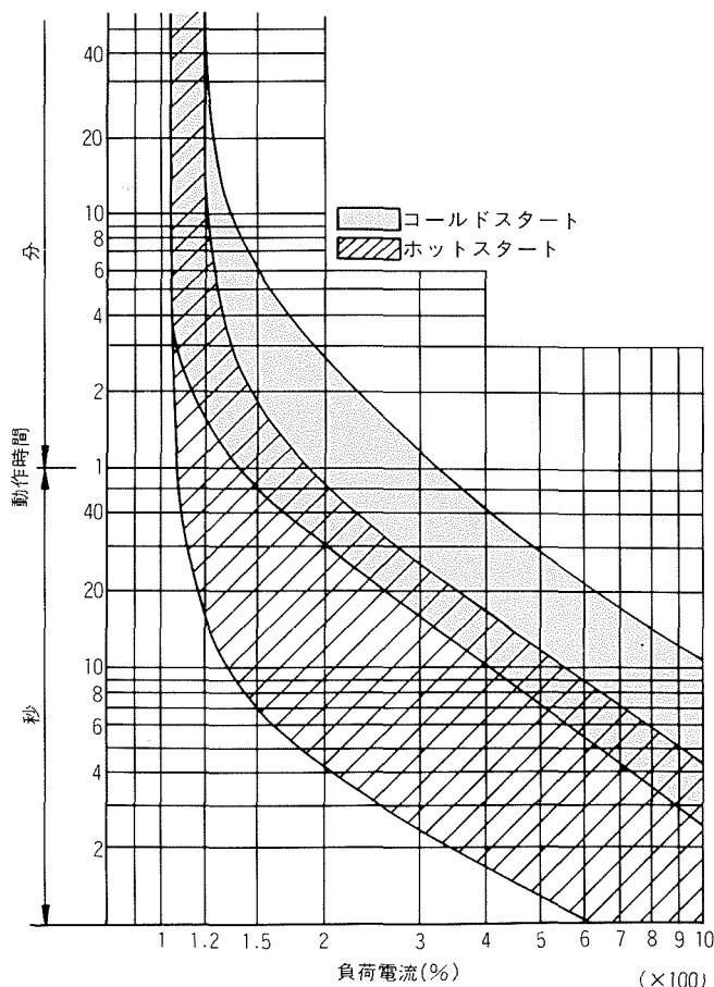
三相過負荷動作特性
