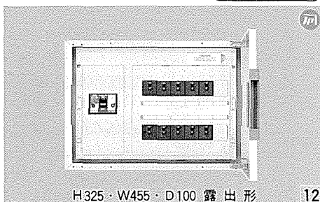
H325・W455・D100 露出形 12
