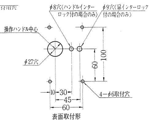
扉穿孔図(扉表面より見た場合)
