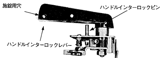
(イ) インターロックをしていない場合
