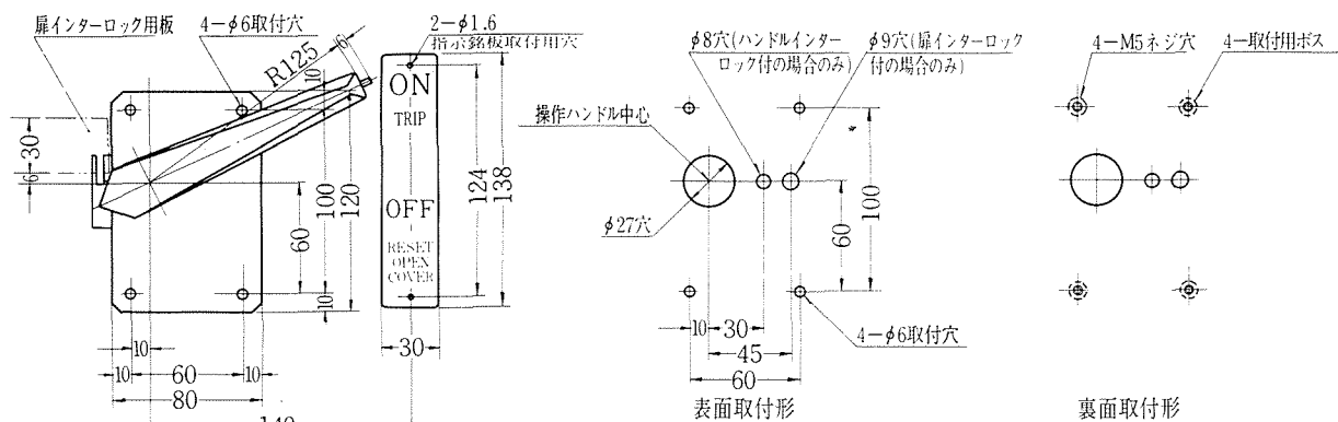
扉穿孔図(扉表面より見た場合)
