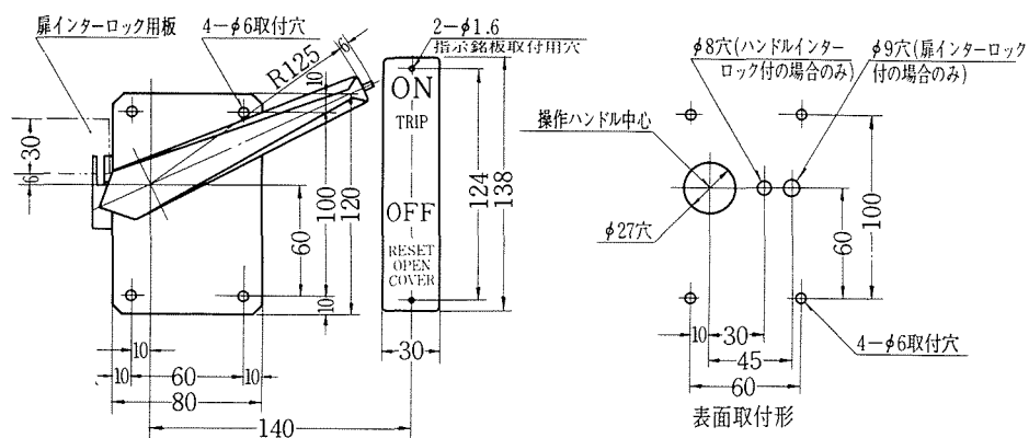
扉穿孔図(扉表面より見た場合)
