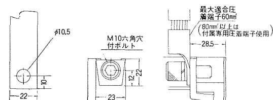
導帯加工図
