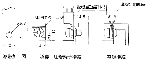
導帯加工図
