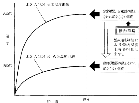
耐熱温度特性
