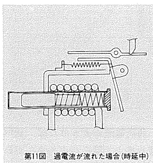
第11図 過電流が流れた場合(時延中)
