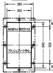
穴明寸法
