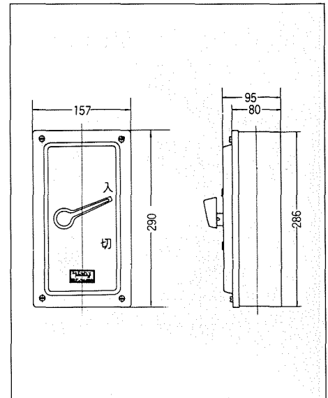
9 DP-BOX
