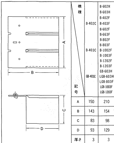
7 端子カバー
