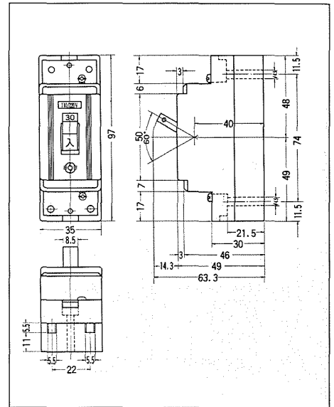
3 JB-32K
