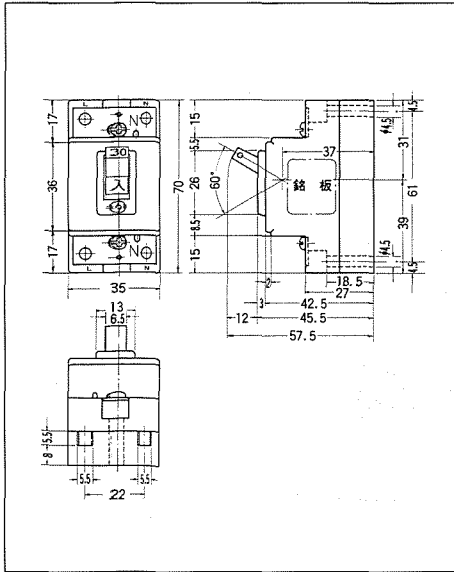
1 JB-1Q・JB-32Q
