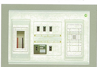
H310・W460・D65 〔主幹〕(ELCB) OCなし 3P30A 100V↔200V相互切替可能
