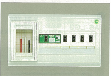
H220・W385・D55 〔主幹〕(ELCB) OCなし 3P30A 100V↔200V相互切替可能
