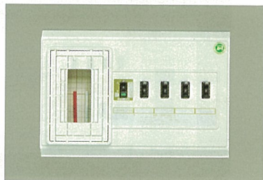
H220・W330・D55 〔主幹〕(ELCB) OCなし 2P30A
