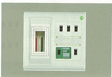
H285・W296・D62 〔主幹〕(ELCB) OCなし 3P30A 100V↔200V相互切替可能
