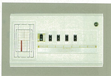
H220・W385・D55 〔主幹〕(ELCB) OCなし 2P30A
