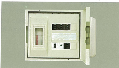
H325・W340・D100 露出形 〔主幹〕(ELCB) OCなし 2P30A
