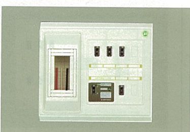
H285・W325・D62 〔主幹〕(ELCB) OCなし 3P30A 100V↔200V相互切替可能
