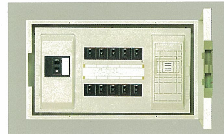
H325・W525・D100 露出形 〔主幹〕(MCB) 3P50A 100V ↔ 200V相互切替可能
