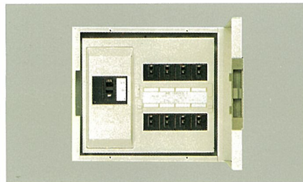
H325・W340・D100 露出形 〔主幹〕(MCB) 3P50A
