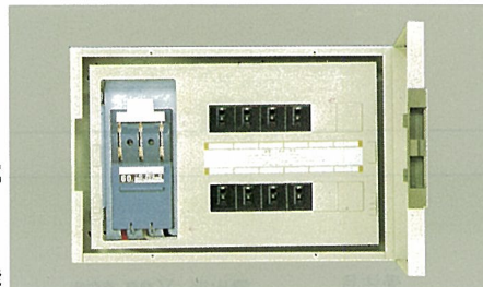
H325・W455・D100 露出形 〔主幹〕(CKS) 3P60A
