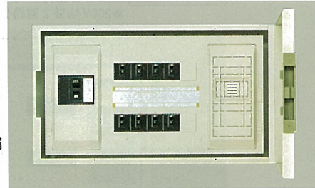
H325・W525・D100 露出形 〔主幹〕(MCB) 3P50A
