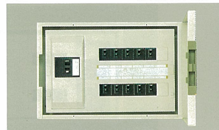
H325・W455・D100 露出形 〔主幹〕(MCB) 3P50A 100V ↔ 200V相互切替可能
