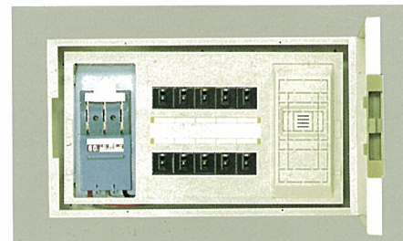
H325・W525・D100 露出形 〔主幹〕(CKS) 3P60A 100V ↔ 200V相互切替可能
