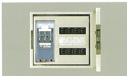
H325・W340・D100 露出形 〔主幹〕(CKS) 3P60A
