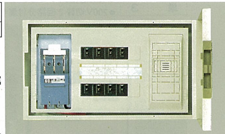
H325・W525・D100 露出形 〔主幹〕(CKS) 3P60A
