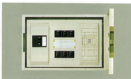
H325・W455・D100 露出形 〔主幹〕 MCB 3P50A
