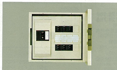
H325・W340・D100 露出形 〔主幹〕 MCB 3P50A 100V ↔ 200V 相互切替可能
