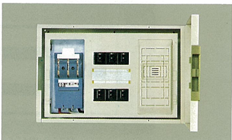
H325・W455・D100 露出形 〔主幹〕 CKS 3P60A 100V ↔ 200V 相互切替可能
