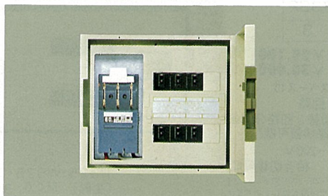
H325・W340・D100 露出形 〔主幹〕 CKS 3P60A 100V ↔ 200V 相互切替可能
