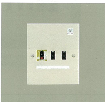
H199・W169・D54 露出形 〔分岐〕 (ELCB) OC付2P20A
