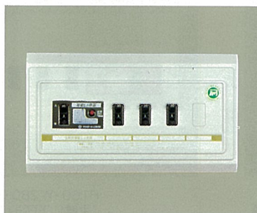
H160・W280・D55 〔主幹〕 (ELCB) OC付2P30A
