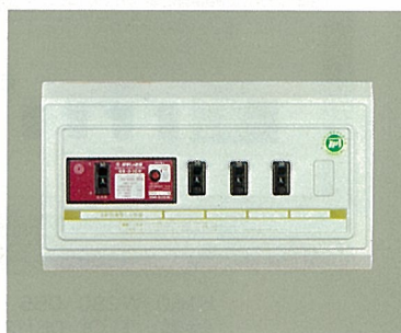
H160・W280・D55 〔主幹〕 (ELCB) OC付3P30A 100V→200V相互切替可能
