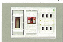
リミッター設置する場合(例)
