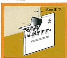
支持板取付け
