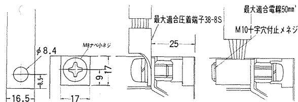
導帯加工図
