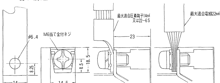
導帶加工図
