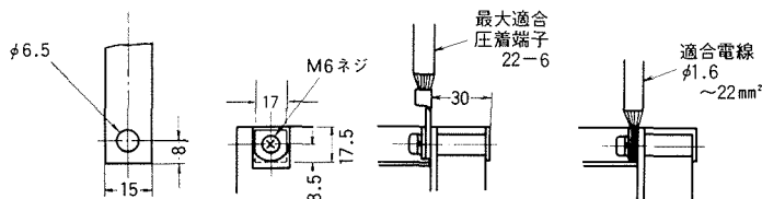
導帯加工図
