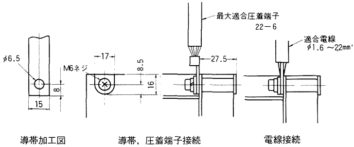
導帯加工図
