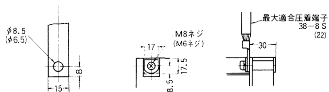
導帯加工図
