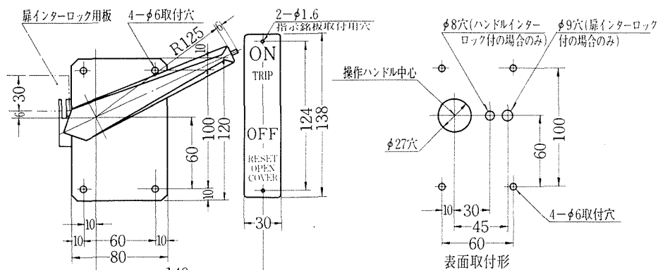
扉穿孔図(扉表面より見た場合)
