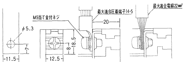
導帯加工図
