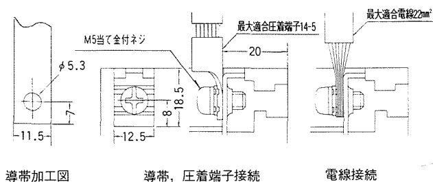
導帯加工図
