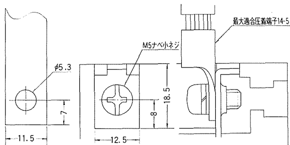
導帯加工図
