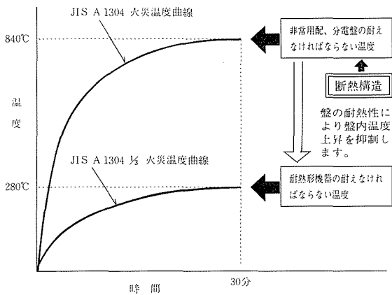
耐熱温度特性
