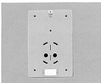
プレート 公団記号V-306-2 ¥1,150 H300・W200・D27
