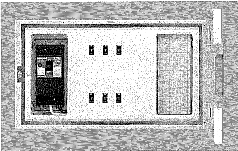
H300・W525・D100 露出形 〔主幹〕 (ELCB) OC付3P40A・50A
