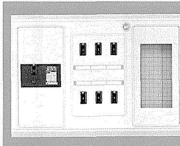
H285・W405・D62 〔主幹〕 (ELCB) OC付3P30A
