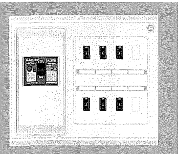
H285・W325・D62 〔主幹〕 (ELCB) OC付3P40A・50A
