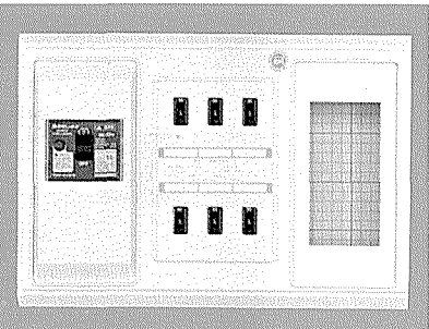
H285・W405・D62 〔主幹〕 (ELCB) OC付3P40A・50A
