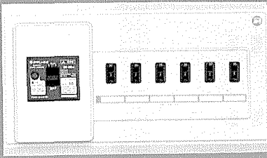
H220・W385・D55 〔主幹〕 (ELCB) OC付3P40A・50A
