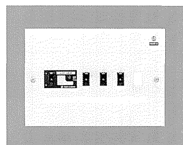
H199・W289・D54 露出形 〔分岐〕 (ELCB) OC付2P20A
