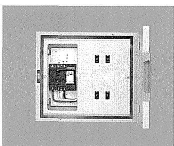
H300・W340・D100 露出形 〔主幹〕 (ELCB) OC付3P30A
