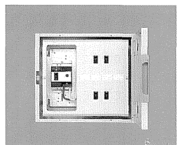
H300・W340・D100 露出形 〔主幹〕 (ELCB) OC付2P30A
