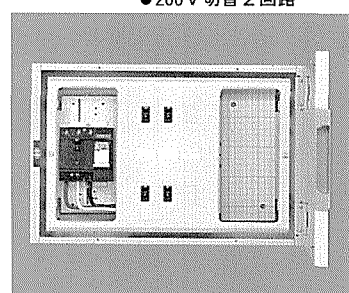
H300・W455・D100 露出形 〔主幹〕 (ELCB) OC付3P30A
