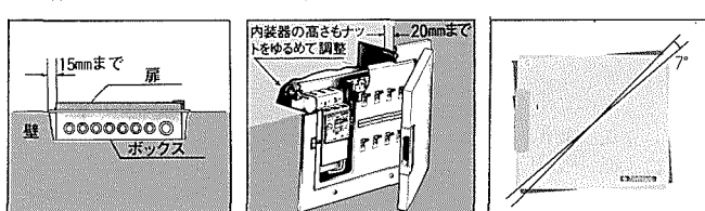
埋込枠
