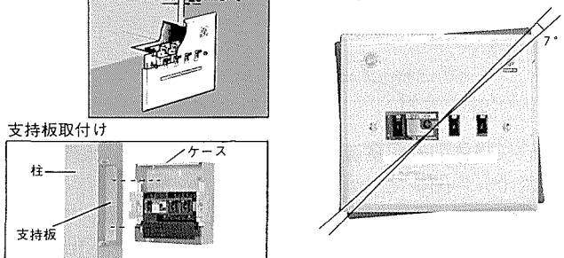
深さ調整
