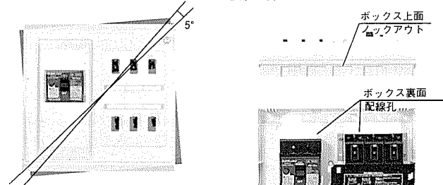
傾き調整
