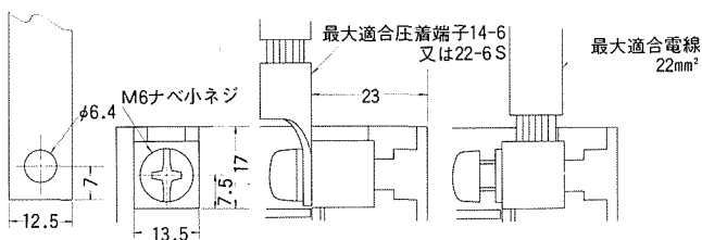
導帯加工図
