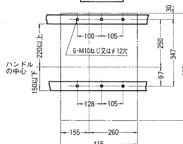
穴明寸法
