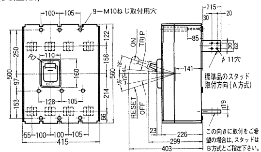
●裏面形(受注品)
