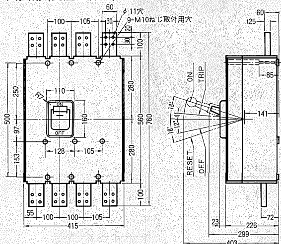
▲埋込形(受注仕様品)
