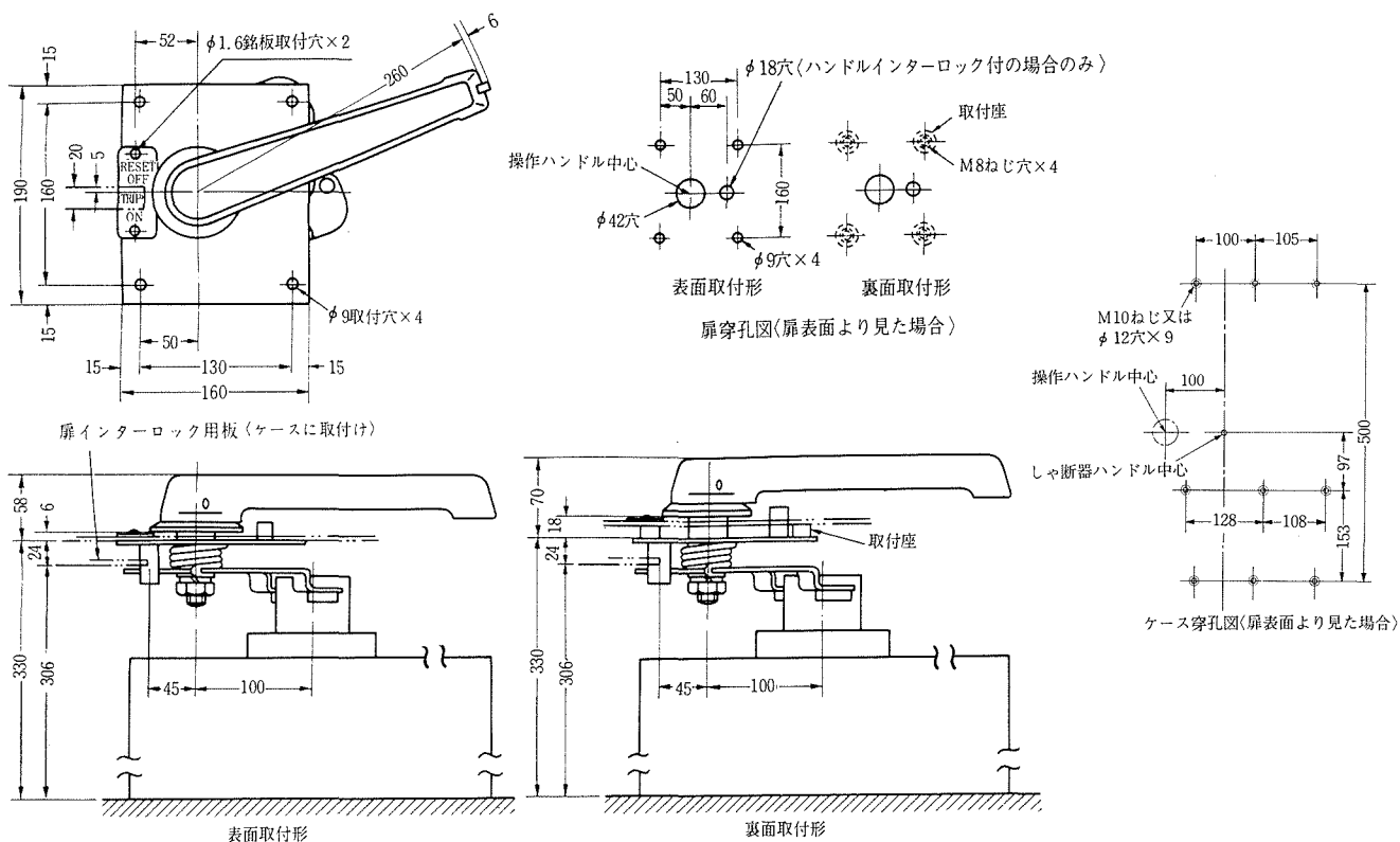
外部操作ハンドル(受注仕様品) 納期別途相談
