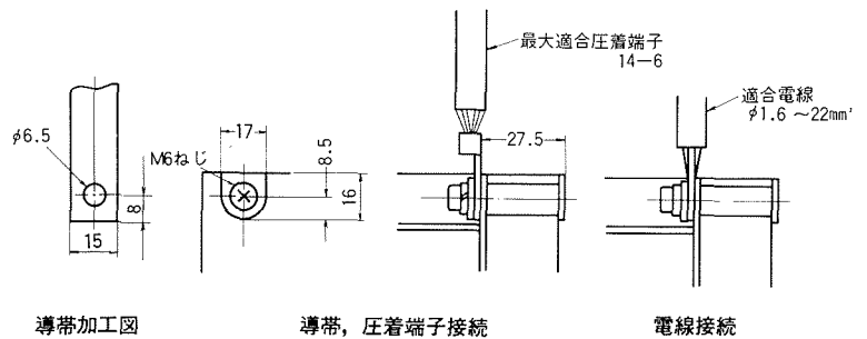
導帯加工図
