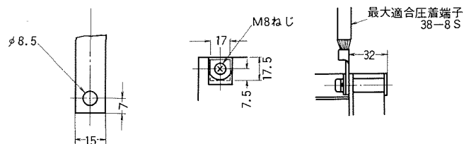
導帯加工図
