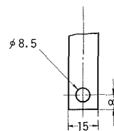
導帯加工図
