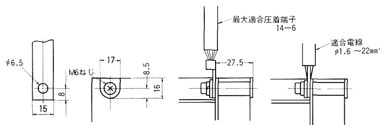
導帯加工図
