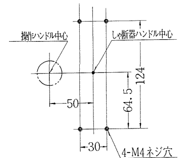
ケース穿孔図(扉表面より見た場合)
