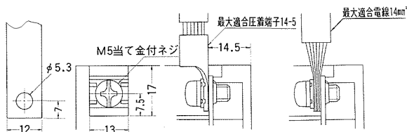
導帯加工図
