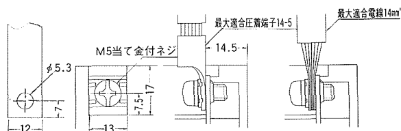
導帯加工図
