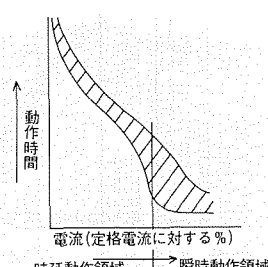
第14図 完全電磁形の動作特性
