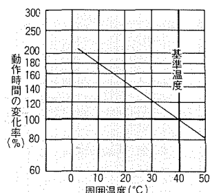
第15図 完全電磁形の温度補正
