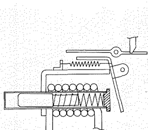
第11図 過電流が流れた場合（時延中）
