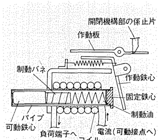
第10図 完全電磁形の原理図
