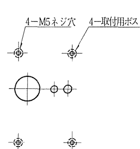
裏面取付形 扉穿孔図(扉表面より見た場合)
