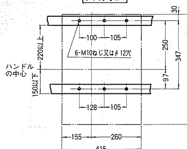
穴明寸法
