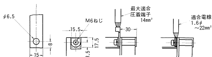
導帯加工図
