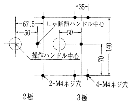
裏面取付形
