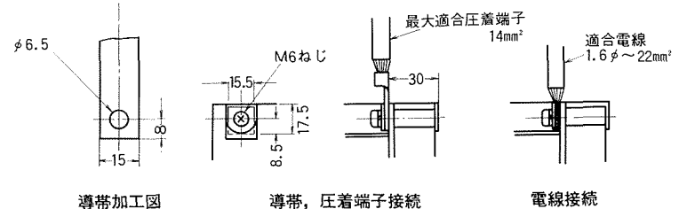
導帯加工図 導帯, 圧着端子接続 電線接続
